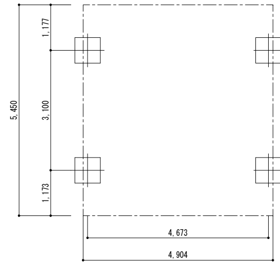
■ 基礎配置図
